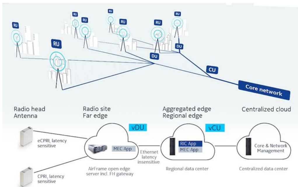
図 2-115G AirScale Cloud RAN のイメージ
