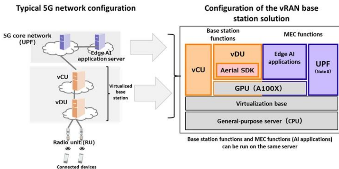
図 2-14NVIDIA5G vRAN ソリューションのイメージ
