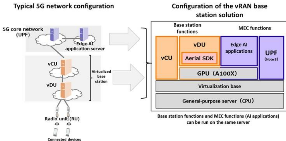
図 3-5 5G 仮想化基地局ソリューションのイメージ
