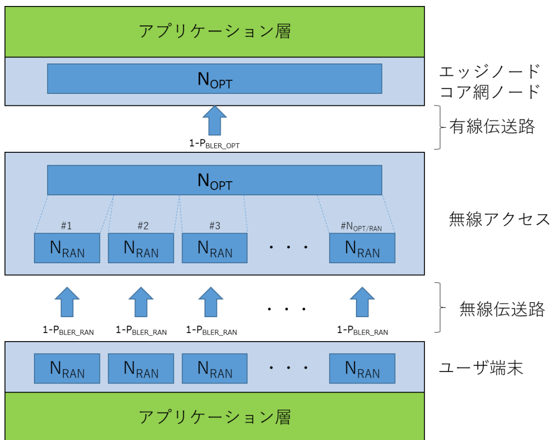
図 5.3-6 エンドツーエンド パケット伝送の簡易検討モデル
