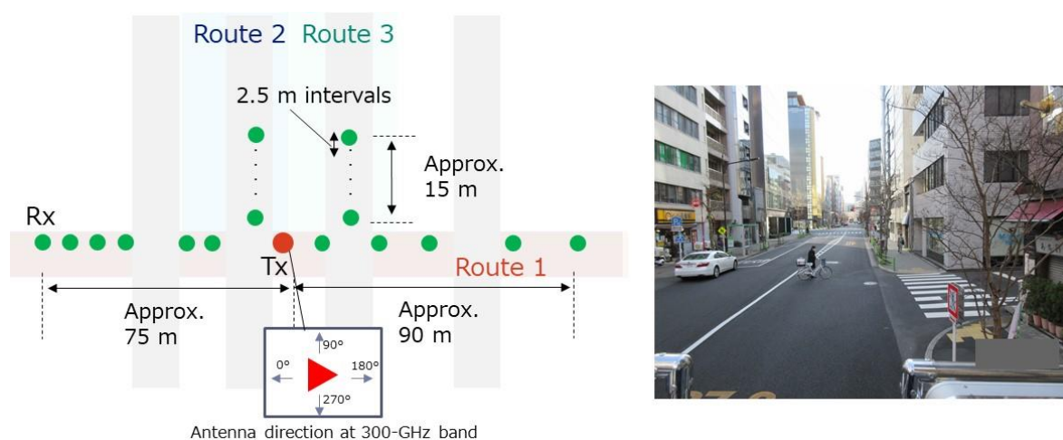
図 6.3-3 市街地マイクロ環境での伝搬損失測定の配置
