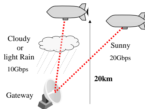
図 6.3-12 100GHz 帯を用いる地上～成層圏のフィーダリンクのシステムモデル
